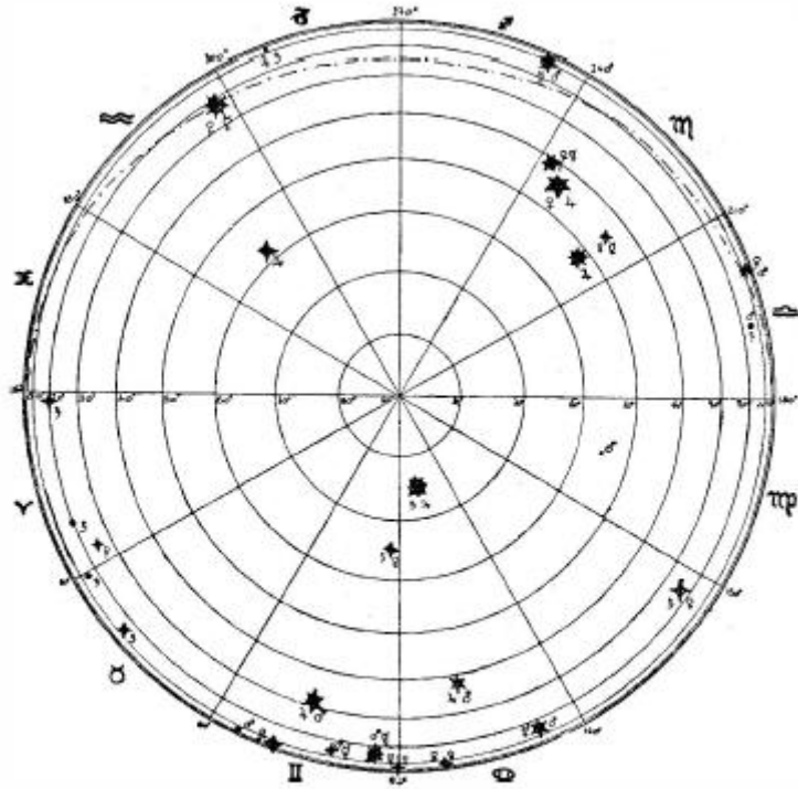
Slunce jižní šíře (—).
