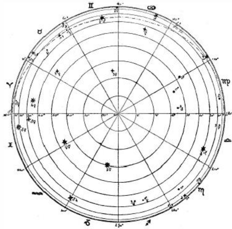
Stálice severní šíře (+).
